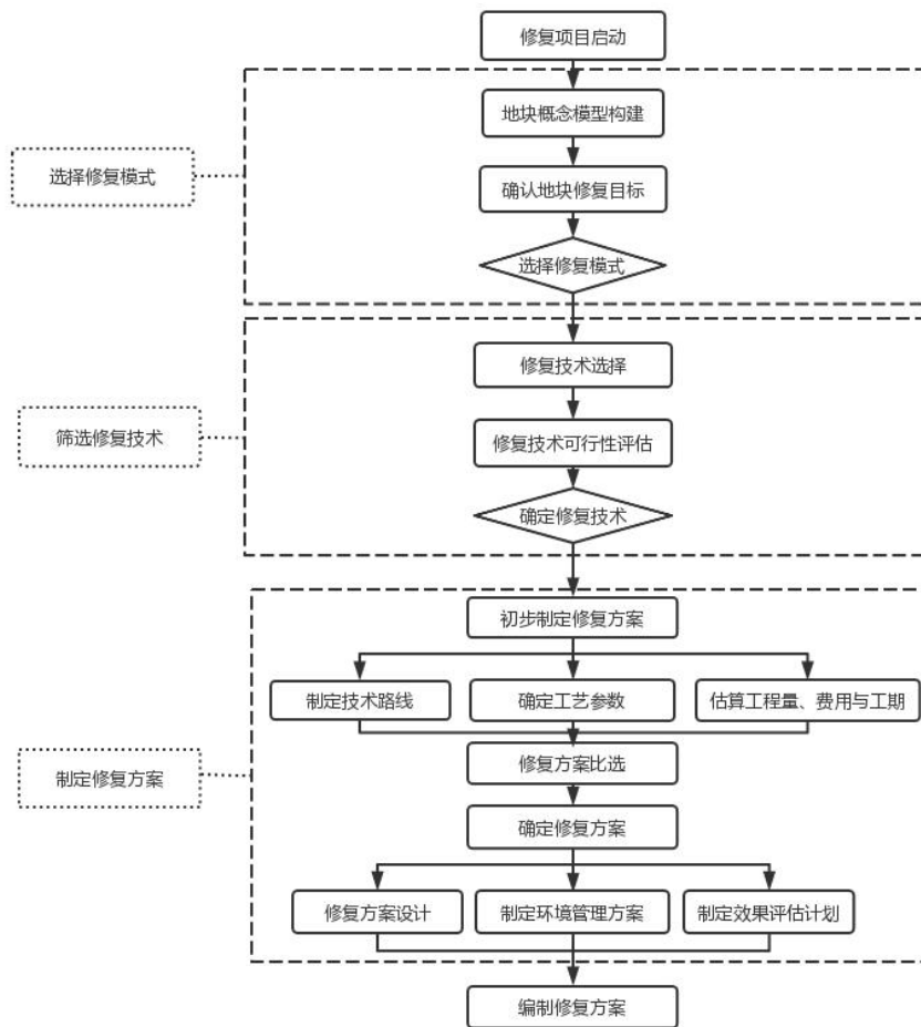
图 1 建设用地土壤污染风险管控和修复方案编制工作程序
